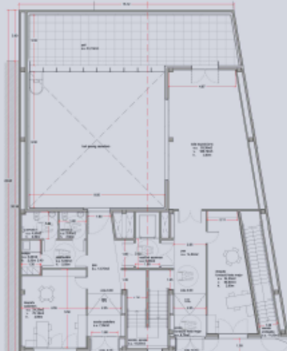
Planta baixa
