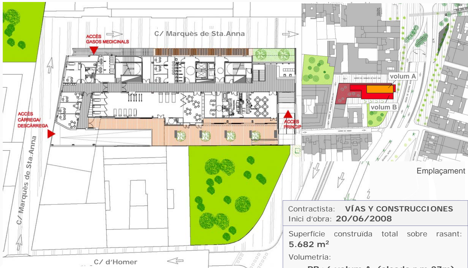
Planta baixa i accessos
