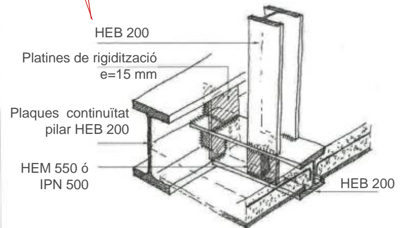
Detall de la unió dels perfils de suport de la façana interior i localització en planta
