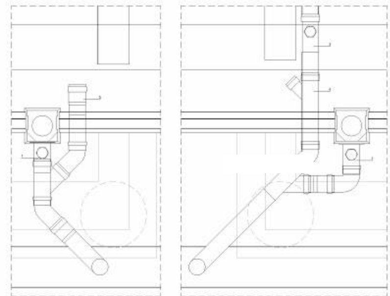
Detalls nou sanejament: connexió a col·lector tipus 1 i tipus 2
