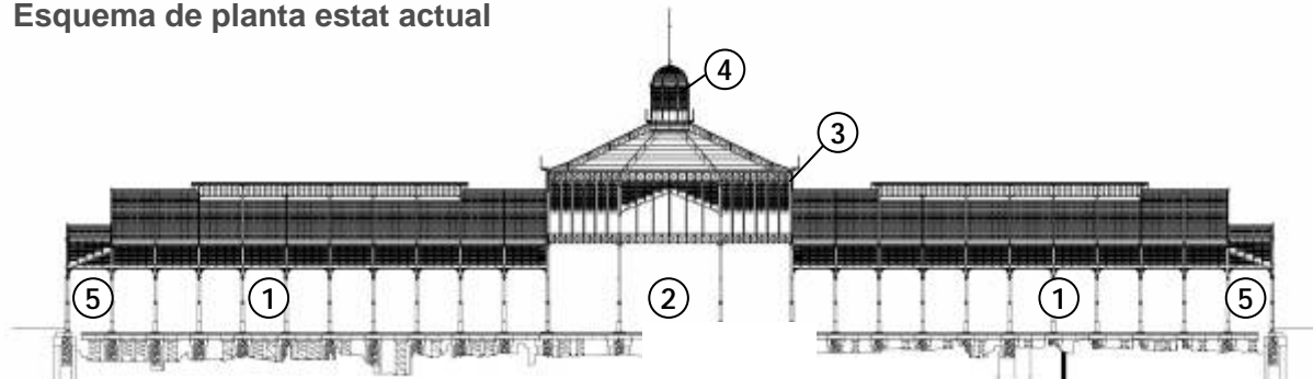
Secció per eix de simetria longitudinal
