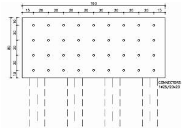
Detail D1. Secció S3 Disposició connectors
