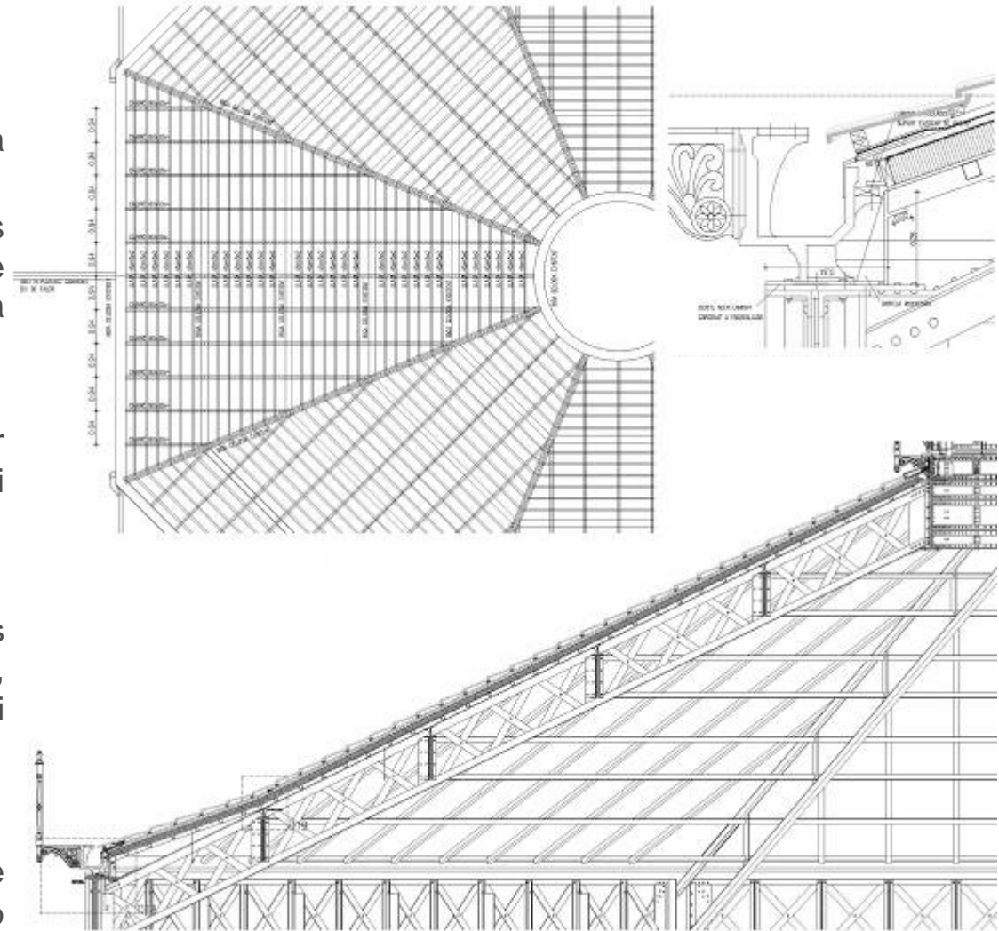
Definició nova estructura de coberta àmbit octògon: planta, secció i detall
