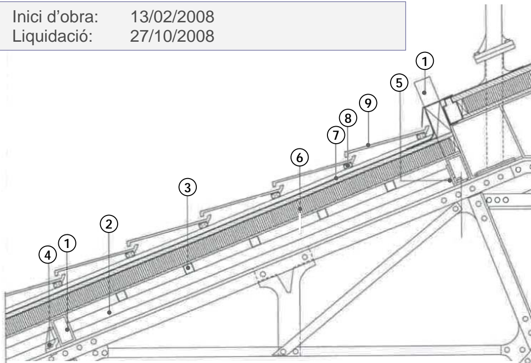
Definició nova estructura de coberta .Detall
