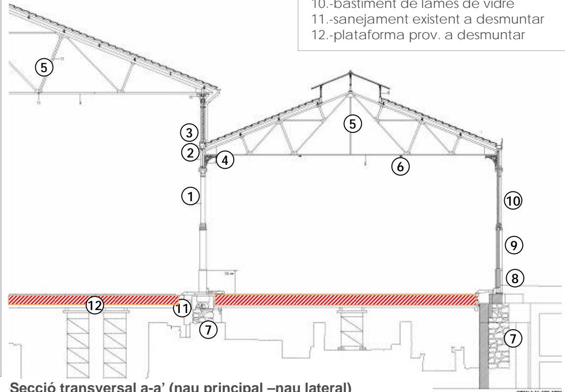
Secció transversal a-a' (nau principal –nau lateral)
