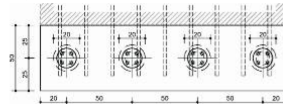
Detail D1. Secció SH1 Situació micropilons en encep
